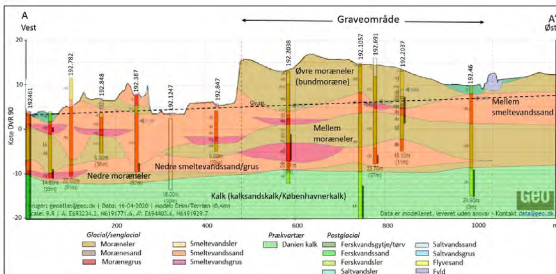
Figur 2: Geologisk profil af foreslået graveområde ved Bøtterup. Det geologiske profil, korreleret med borer i området, viser at der kun er en lille og dybtliggende ressource af sand i det foreslåede graveområde. Forslag til graveområde Bøtterup forkastes derfor.
