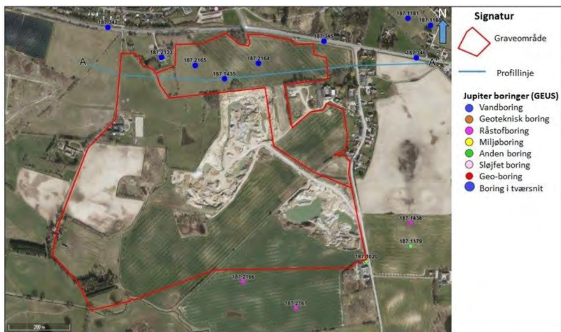
Figur 3: Graveområde med profilinje og borer. De store blå markeringer er de borer, der indgår i den geologiske tolkning af tværsnittet (figur 2).
