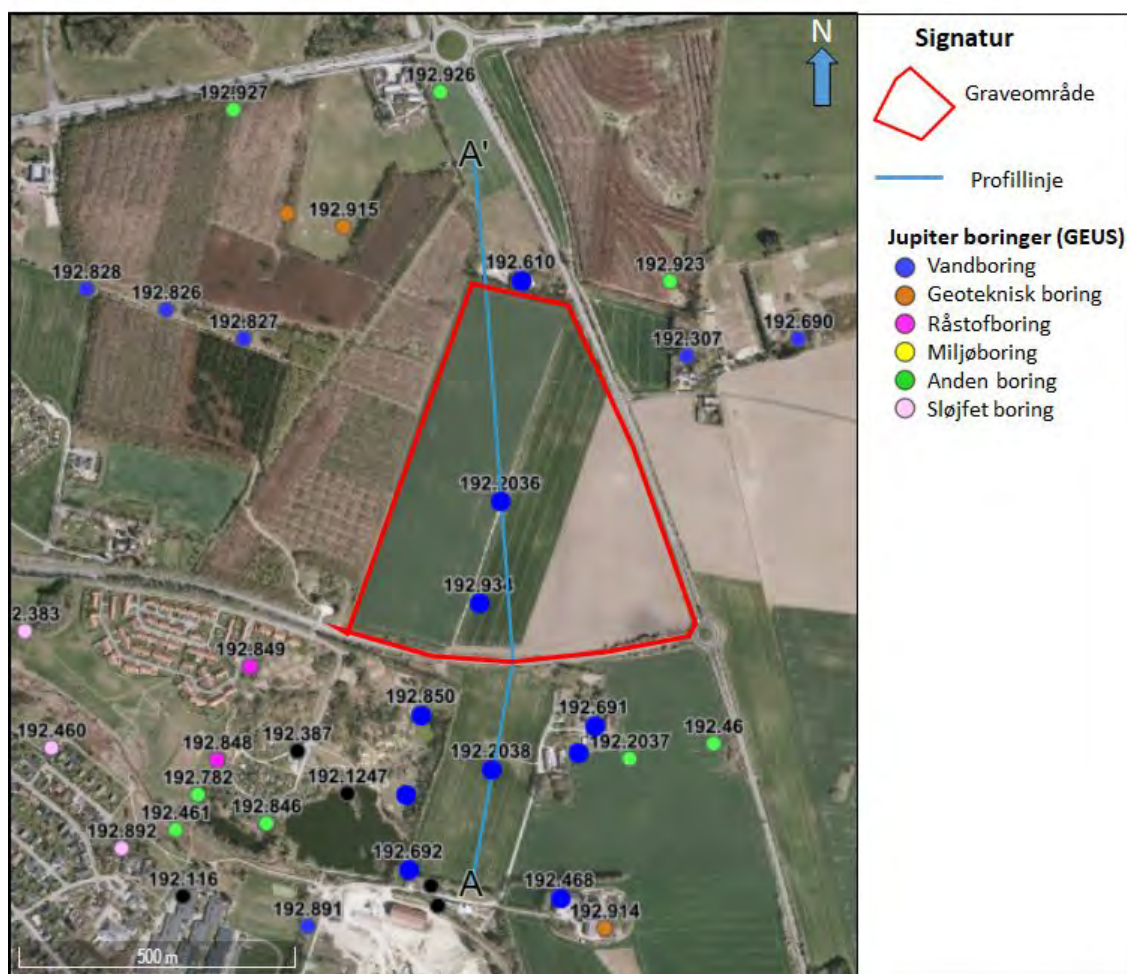
Figur 3: Graveområde med profillinje og borer. De store blå markeringer er de borer, der indgår i den geologiske tolkning af tværsnittet (figur 2).
