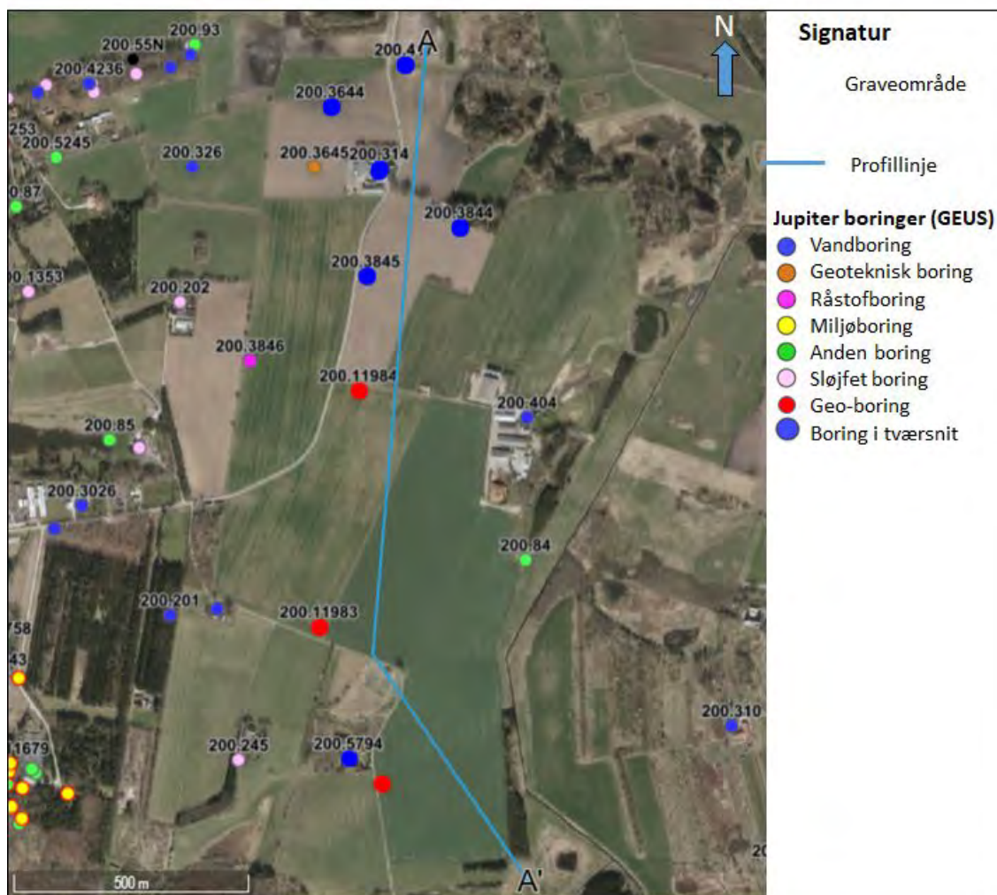
Figur 3: Graveområde med profillinje og borer. De store blå markeringer er de borer, der indgår i den geologiske tolkning af tværsnittet (figur 2)
