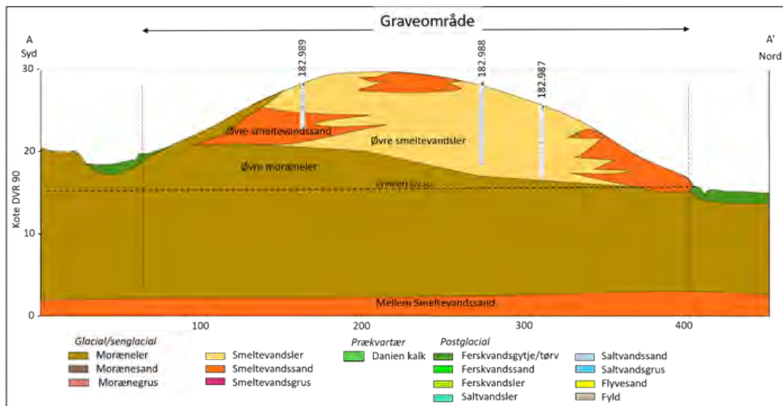
Figur 4. Geologisk tværsnit af graveområde 3 Blistrup med tolket geologisk lagfølge i området. Profilinjens placering fremgår af figur 5.
