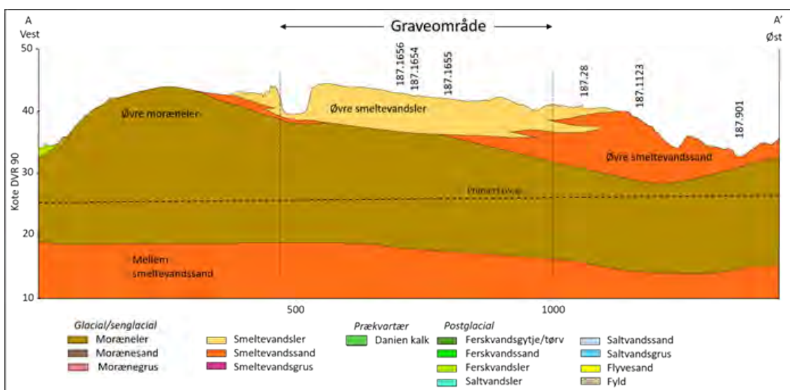
Figur 2. Geologisk tværsnit for graveområde 10 Mårum med tolket geologisk lagfølge i området. Profilinjens placering fremgår af figur 3.
