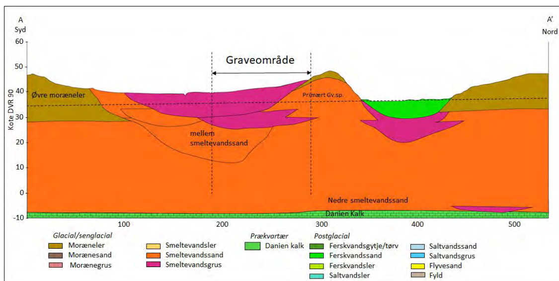
Figur 2: Geologisk tværsnit med tolket geologisk lagfølge i området. Profilinjen placeret fremgår af figur 3.
