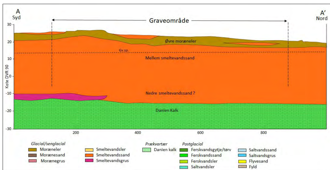
Figur 2: Geologisk tværsnit med tolket geologisk lagfølge i området. Profillinjen placering fremgår af figur 3.
