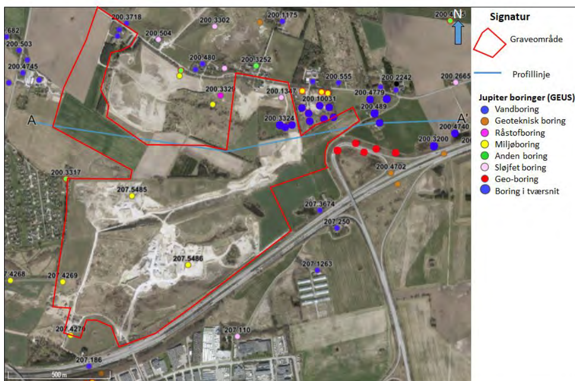
Figur 3: Graveområde med profilinje og borer. De store blå markeringer er de borer, der indgår i den geologiske tolkning af tværsnittet (figur 2).
