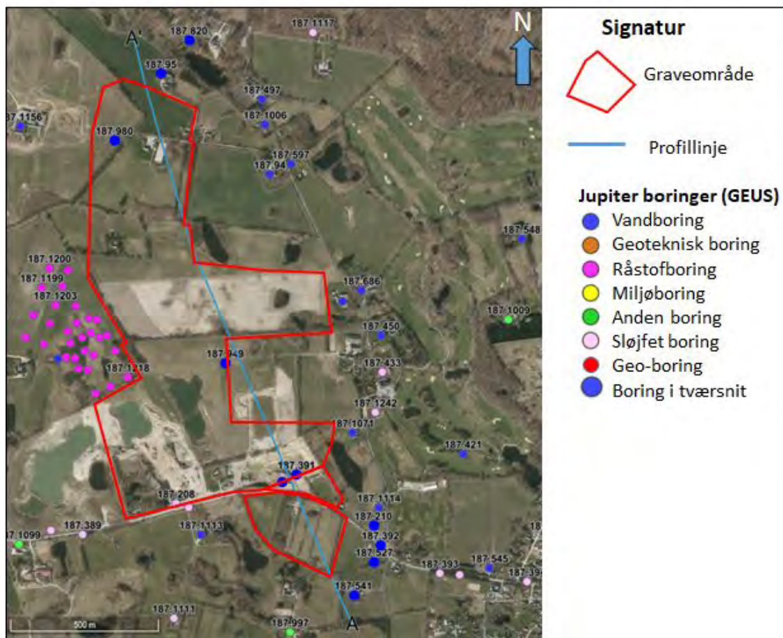
Figur 3: Graveområde med profillinje og boringer. De store blå markeringer er de boringer, der indgår i den geologiske tolkning af tværsnittet (figur 2).
