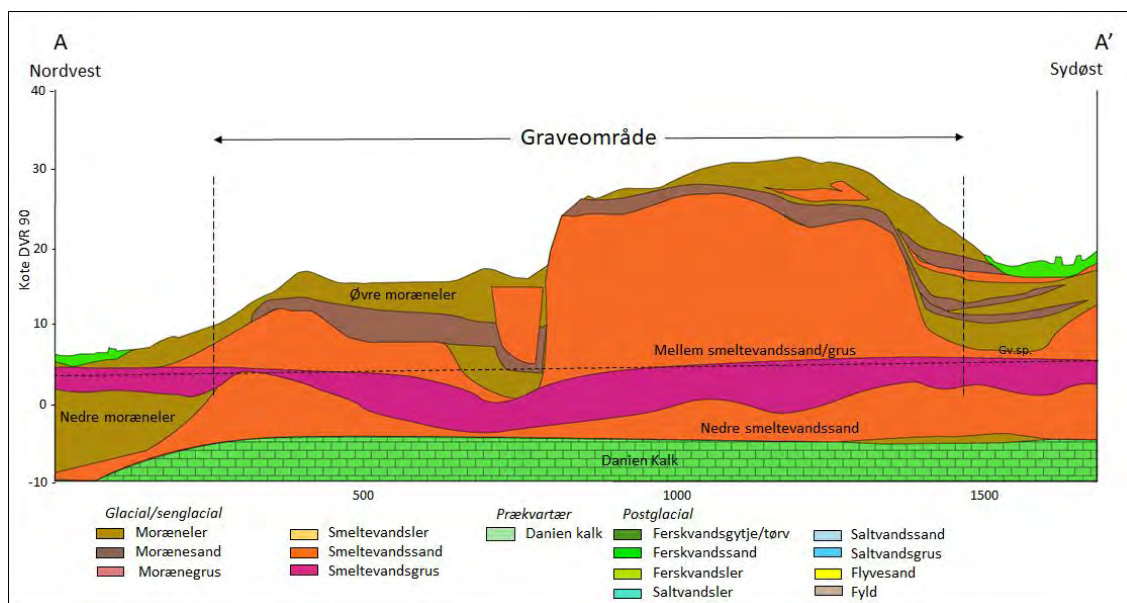
Figur 2: Geologisk tværsnit med tolket geologisk lagfølge i området. Profilinjen
