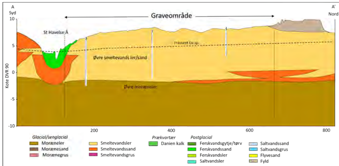
Figur 2. Geologisk tværsnit med tolket geologisk lagfølge i graveområde 22 og 23. Profillinjens placering fremgår af figur 3.
