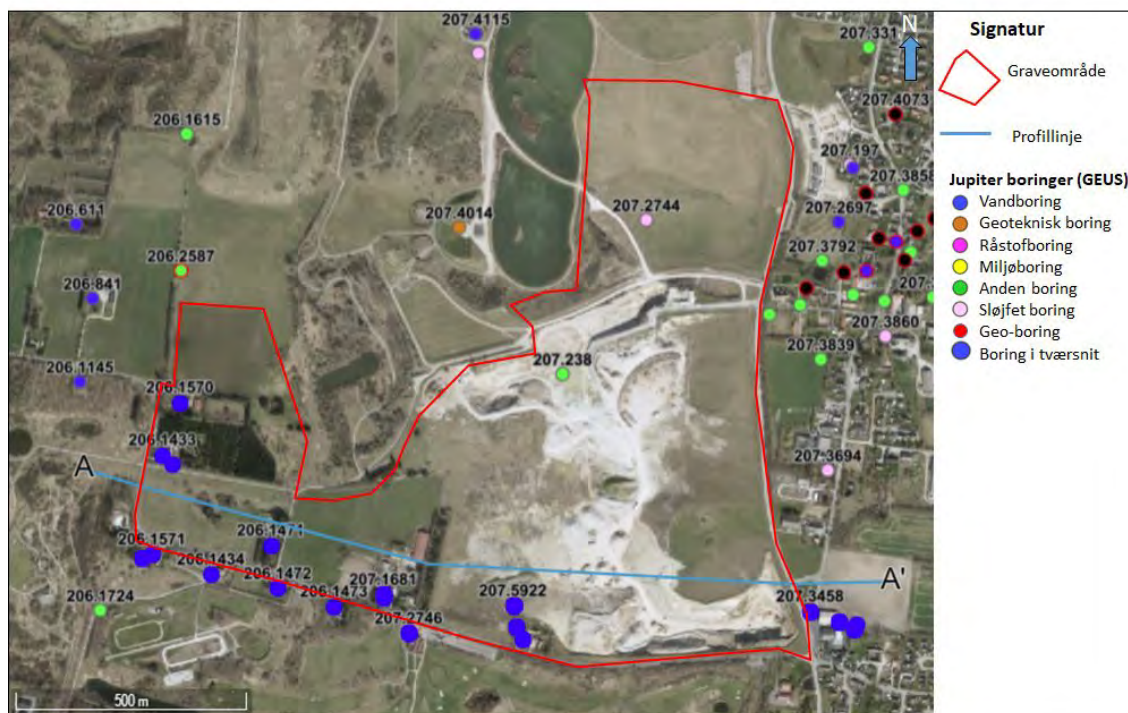
Figur 3: Graveområde med profilinje og boringer. De store blå markeringer er de boringer, der indgår i den geologiske tolkning af tværsnittet (figur 2). Afgrænsningen af graveområdet er den afgrænsning området havde i Råstofplan 2012. Afgrænsningen er reduceret i Råstofplan 2016/2020 (figur 1).
