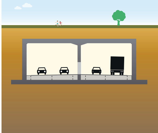
Figur 9: Nedgravet tunnel.
