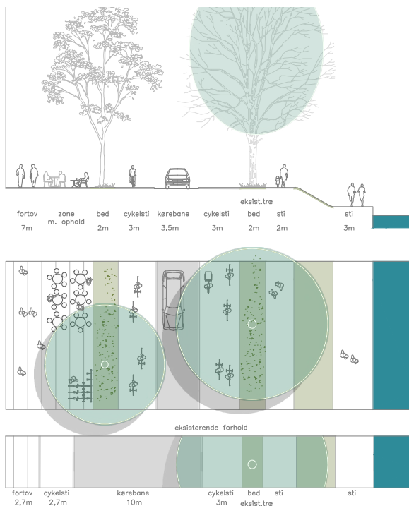
Figur 24: Principsnit og plantegning for en mulig fremtidig udformning af Nørre Søgade. Tegninger: LYTT Architecture.
