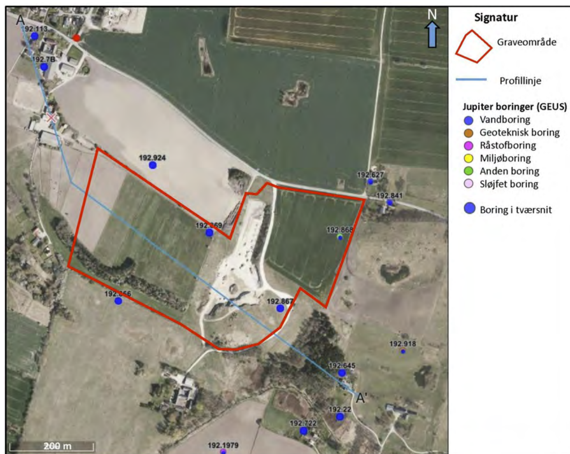
Figur 3: Afgrænsning af graveområde med profillinje og borer. De store blå markeringer er de borer, der indgår i den geologiske tolkning af tværsnittet (figur 2).
