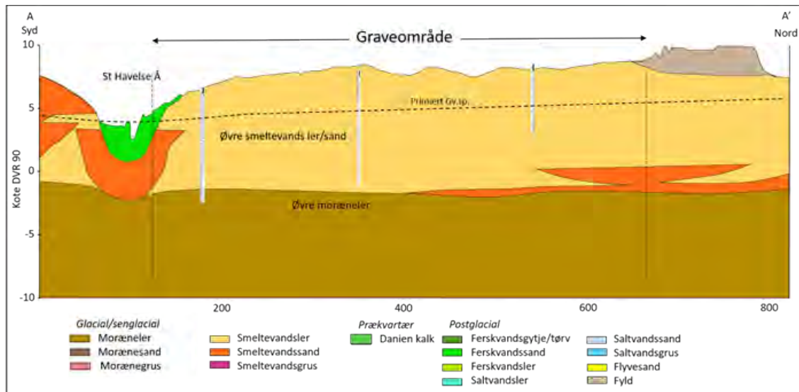
Figur 2. Geologisk tværsnit med tolket geologisk lagfølge i graveområde 22 og 23. Profilinjen placering fremgår af figur 3.
