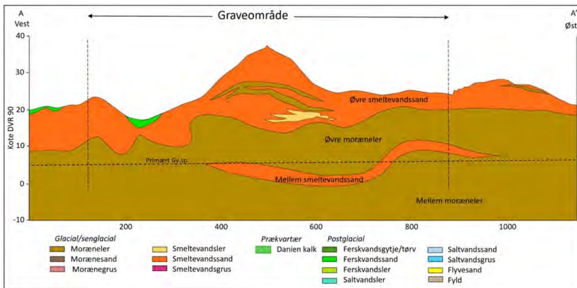
Figur 2: Geologisk tværsnit med tolket geologisk lagfølge i området. Profilinjen placering fremgår af figur 3.
