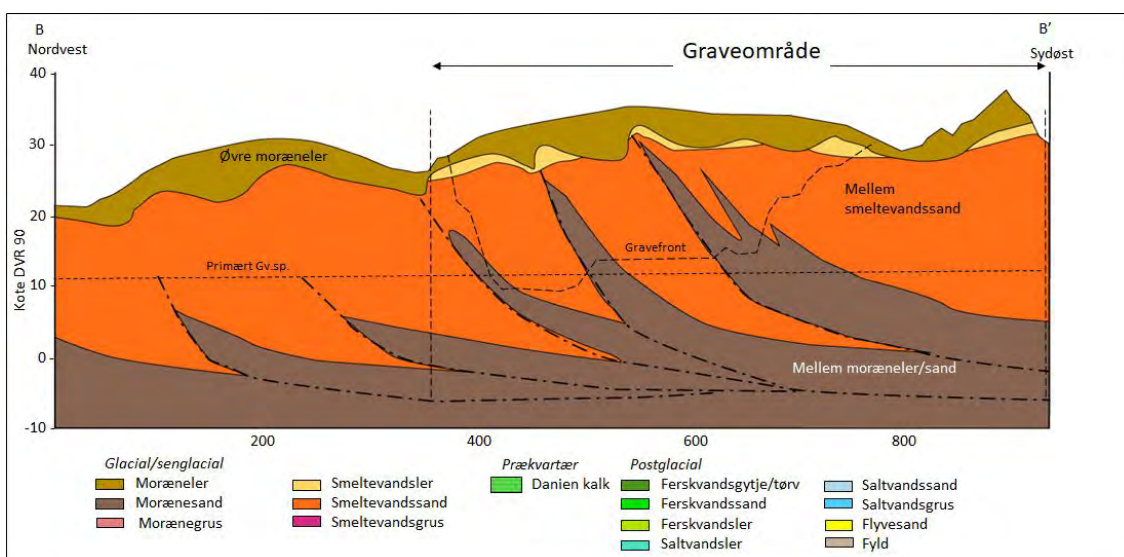
Figur 3: Geologisk tværsnit B-B' med tolket geologisk lagfølge i området.
