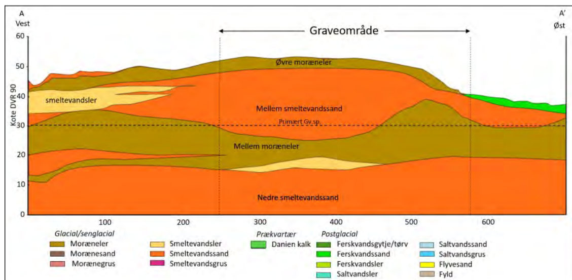
Figur 4 Geologisk tværsnit med tolket lagfølge i den del af A4 Kvistgård udlagt i 2025 (tidl. Kvistgård Udv.). Profillinjen placering fremgår af figur 5.
