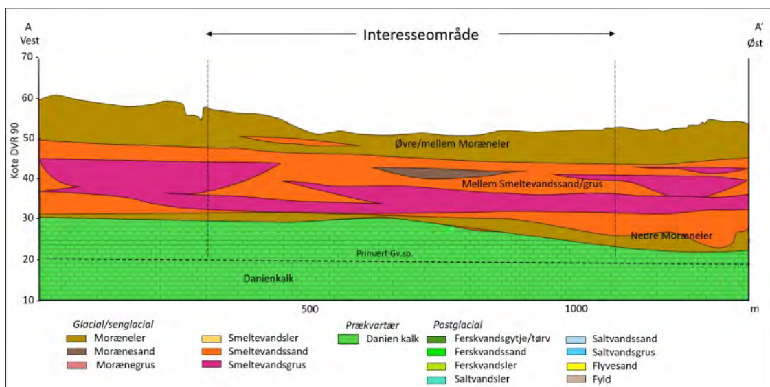
Figur 2. Geologisk tværsnit med tolket lagfølge i området J6 Stærkende. Profilets placering fremgår af figur 3.
