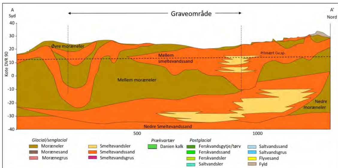
Figur 2. Geologisk tværsnit med tolket lagfølge i graveområde K1 Holtegård. Profillets placering fremgår af figur 3.
