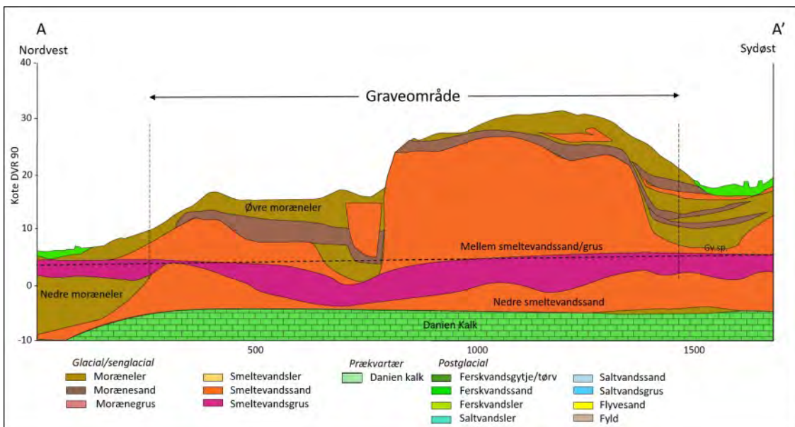
Figur 2. Geologisk tværsnit med tolket lagfølge i graveområdet D10 Lille Rørbæk. Profilets placering fremgår af figur 3.
