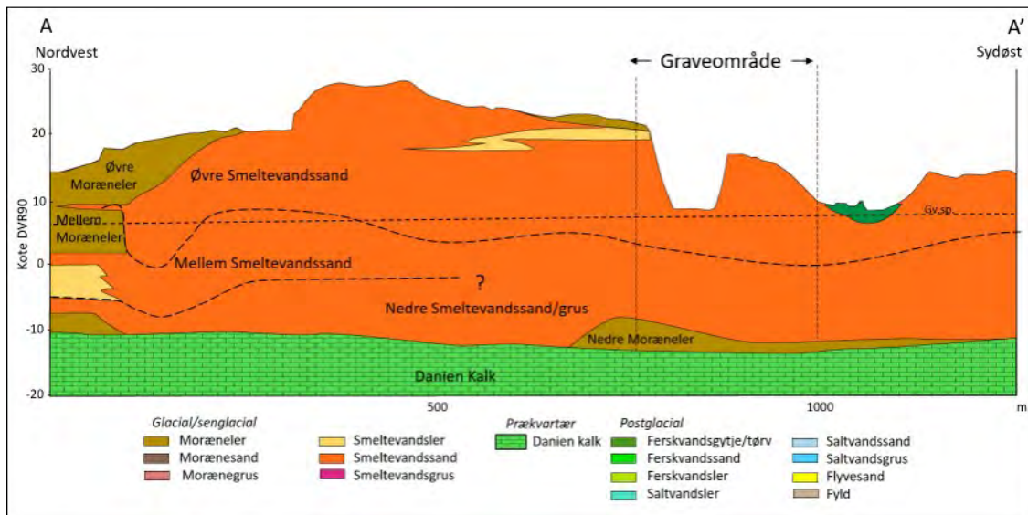
Figur 2. Geologisk tværsnit med tolket lagfølge i graveområdet D7 Ryegård. Profilets placering fremgår af figur 3.
