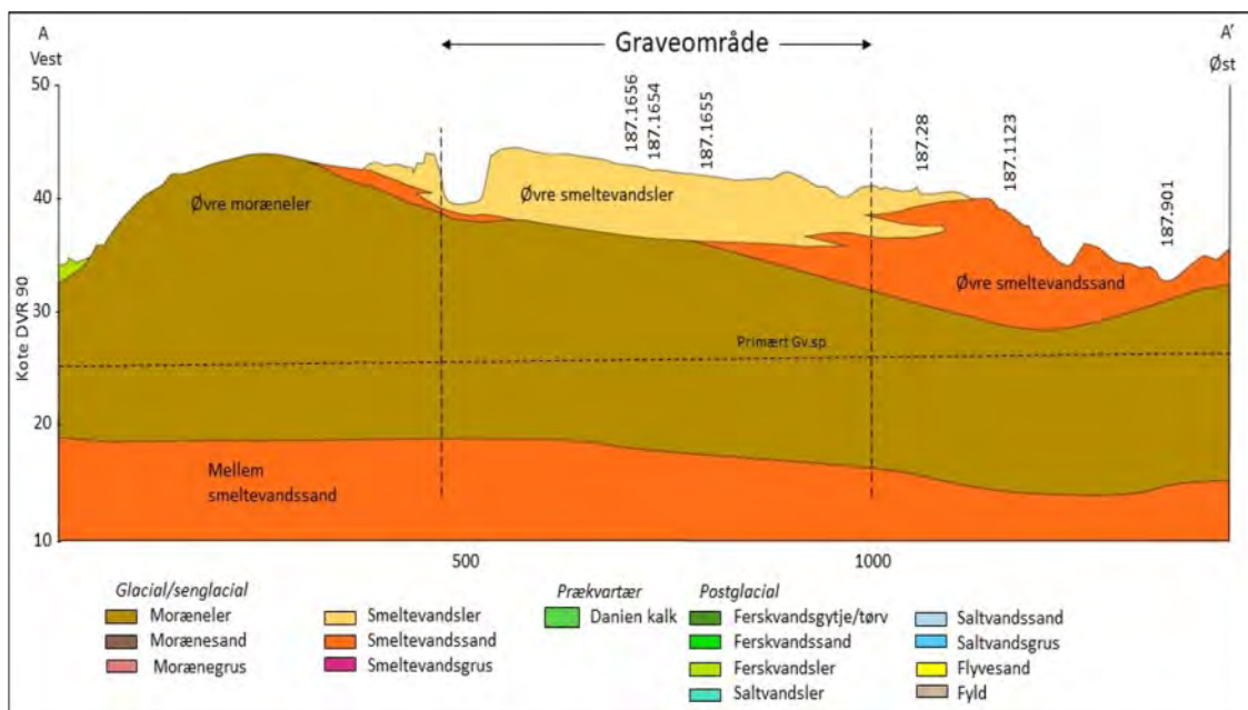
Figur 2. Geologisk tværsnit med tolket lagfølge i området 7 Dønnevælde. Profillets placering fremgår af figur 3.
