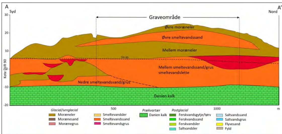
Figur 2. Geologisk tværsnit med tolket lagfølge i graveområdet D9 Grønlien. Profillets placering fremgår af figur 3.
