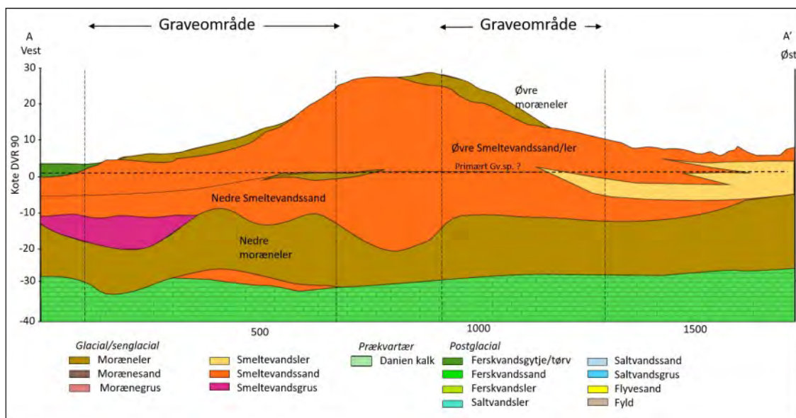
Figur 2. Geologisk tværsnit med tolket geologisk lagfølge i graveområdet C5 Amager Huse. Profilinjens placering fremgår af figur 3.
