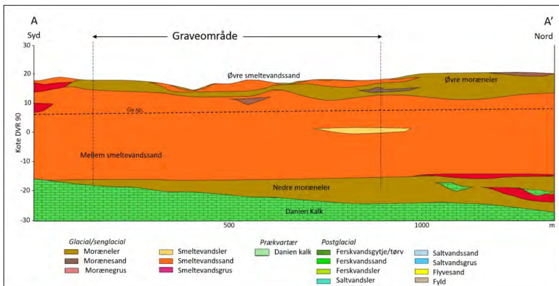
Figur 2. Geologisk tværsnit med tolket lagfølge i graveområdet D8 Landerslev Vest. Profilets placering fremgår af figur 3.
