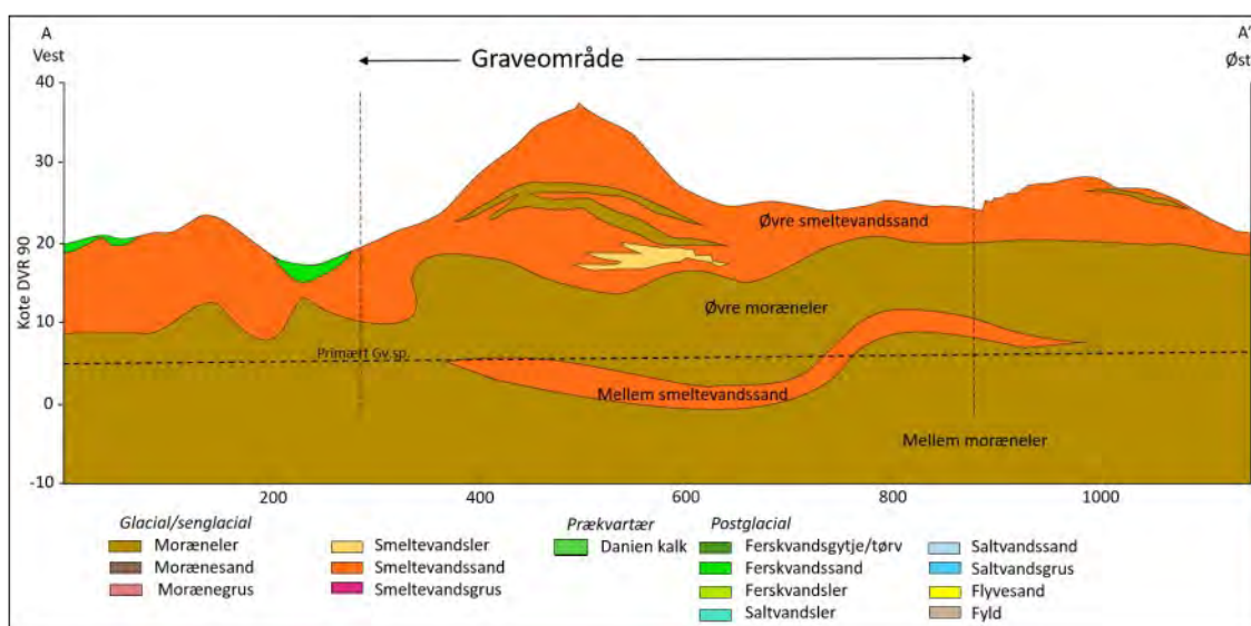
Figur 2. Geologisk tværsnit med tolket geologisk lagfølge i området B1 Ammendrup. Profilinjens placering fremgår af figur 3.
