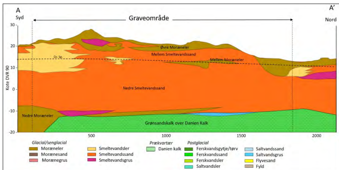
Figur 2. Geologisk tværsnit med tolket lagfølge i graveområdet D11 Onsved. Profilets placering fremgår af figur 3.
