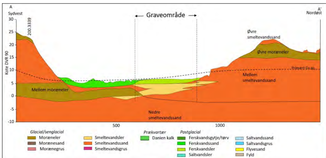
Figur 2 Geologisk tværsnit med tolket lagfølge i området 28 Knardrup. Profilets placering fremgår af figur 3.
