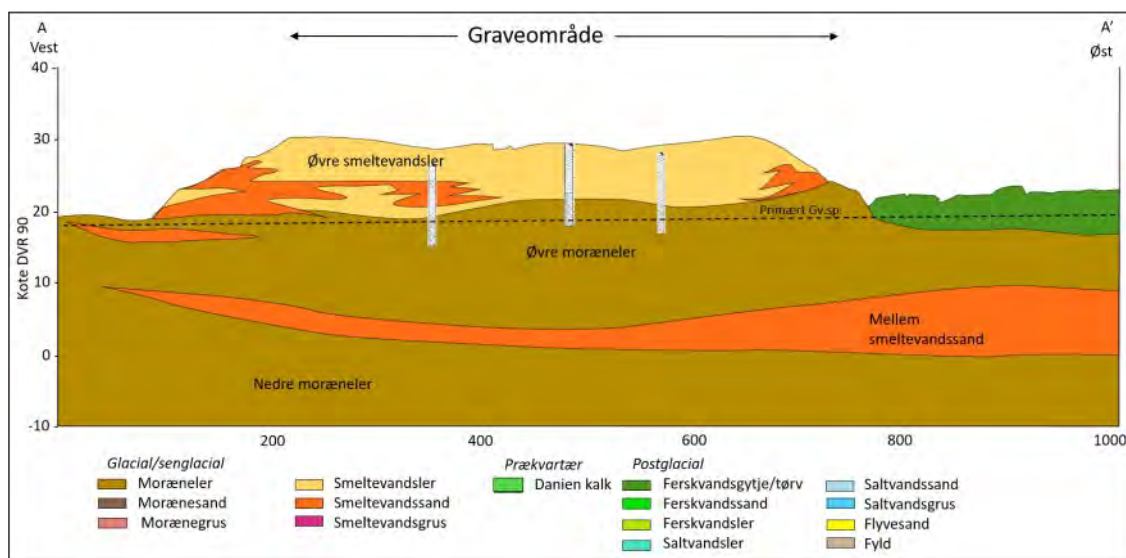
Figur 2. Geologisk tværsnit med tolket lagfølge i området 10 Nellerød. Profilets placering fremgår af figur 3.
