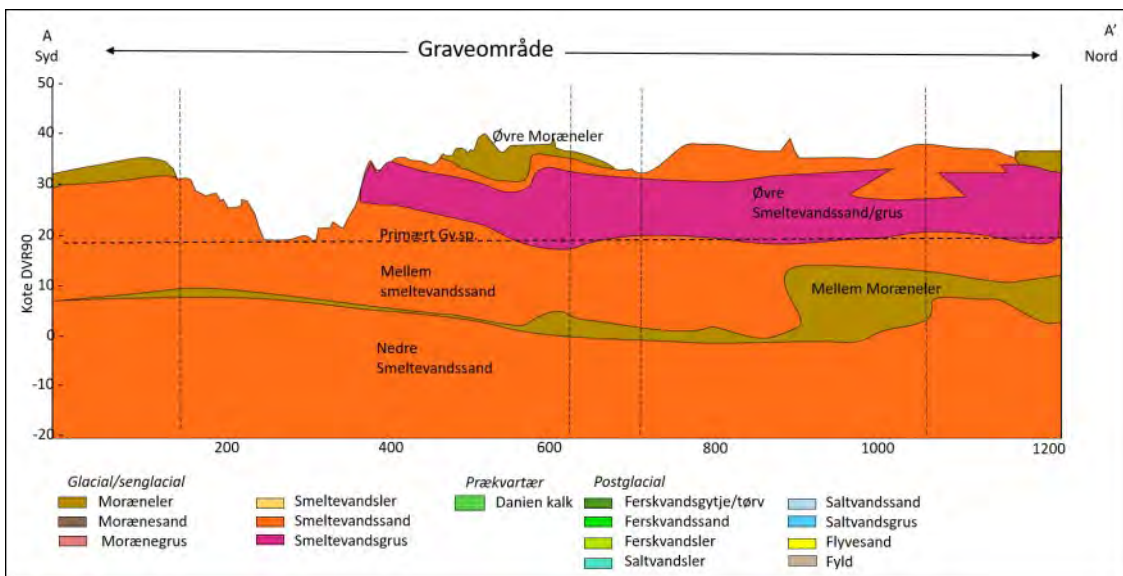
Figur 2. Geologisk tværsnit med tolket geologisk lagfølge i området A1 Bøtterup. Profillinjens placering fremgår af figur 3.
