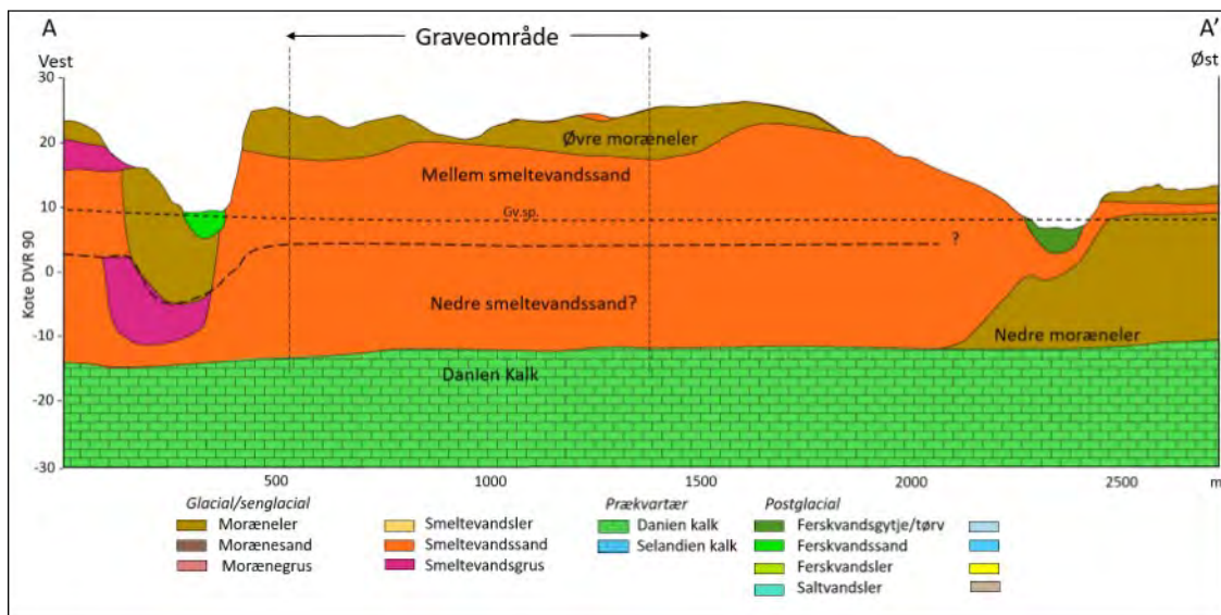
Figur 2. Geologisk tværsnit med tolket lagfølge i området D6 Kyndby - del udlagt i 2007. Profillets placering fremgår af figur 3.
