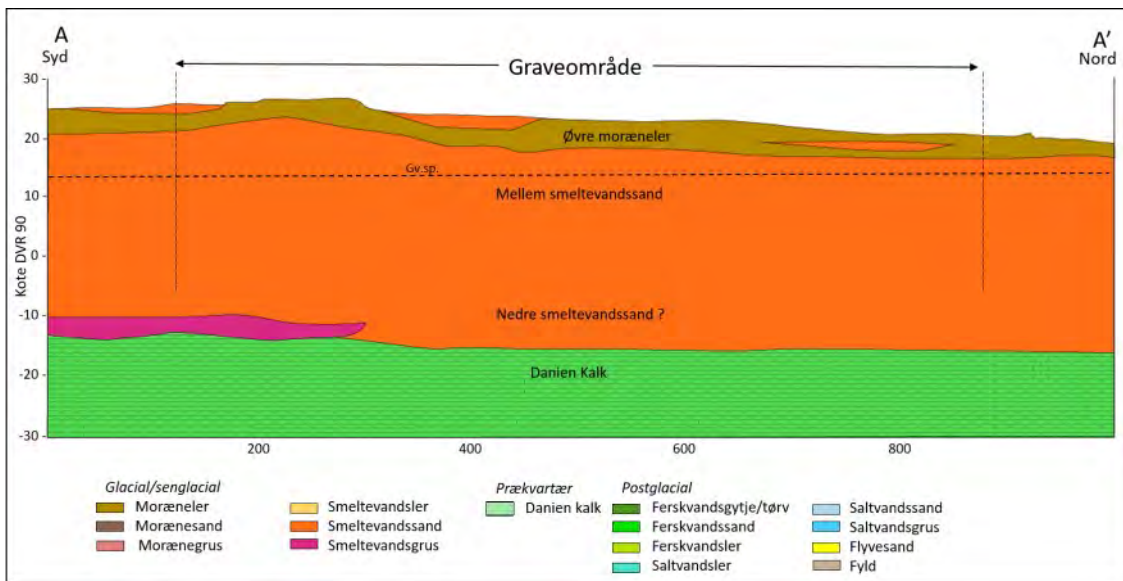
Figur 2. Geologisk tværsnit med tolket lagfølge i graveområdet D12 Krogstrup. Profilets placering fremgår af figur 3.
