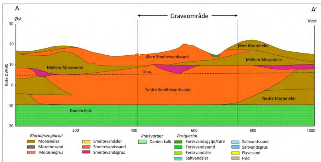
Figur 4. Geologisk tværsnit med tolket geologisk lagfølge i området D2 Sundbylille - del udlagt i 2025 (tidl. Sundbylille udv.). Profilinjen's placering fremgår af figur 5.
