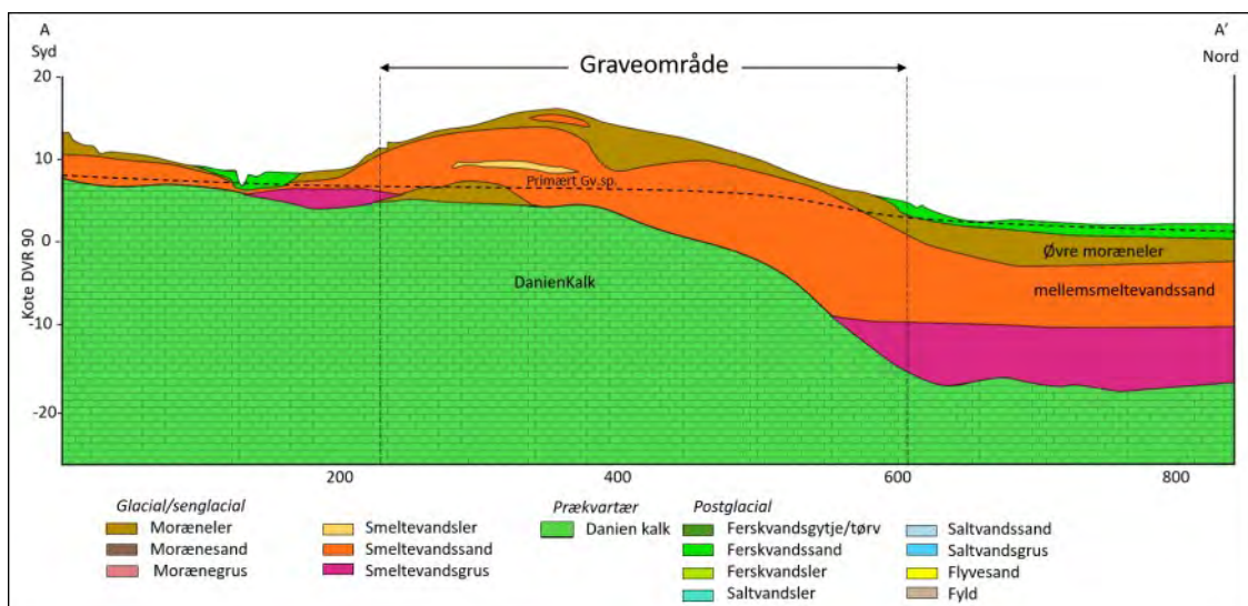
Figur 2. Geologisk tværsnit med tolket lagfølge i graveområdet L3 Hove Møllevej. Profilets placering fremgår af figur 3.
