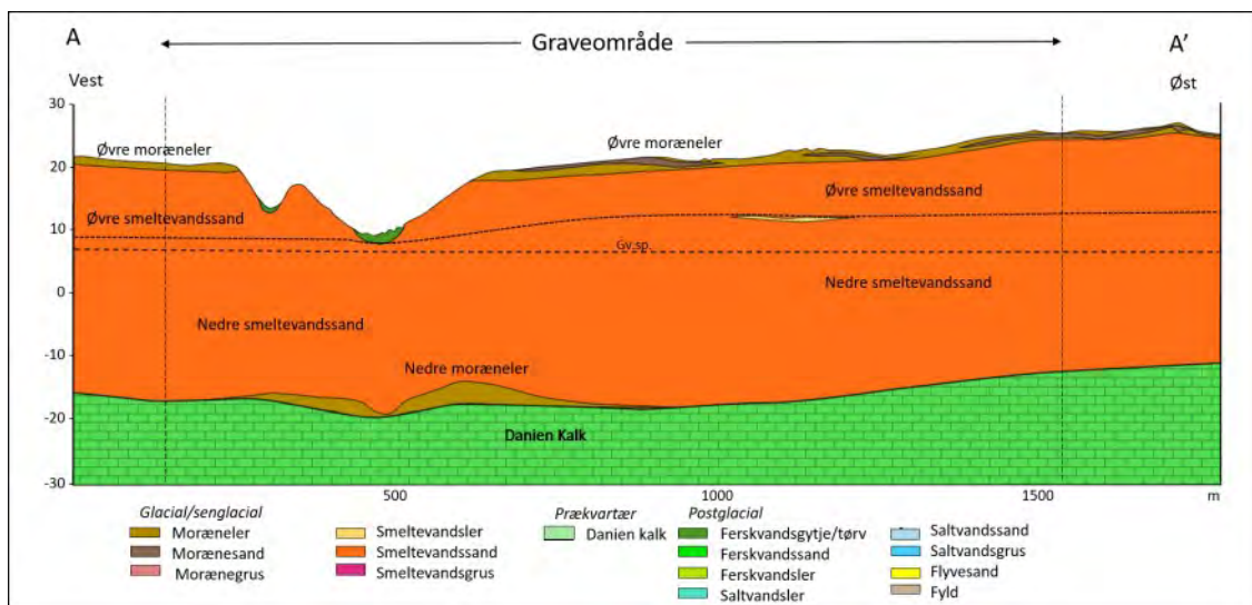
Figur 4. Geologisk tværsnit med tolket lagfølge i området D6 Kyndby - del udlagt i 2025 (tidl. Kyndby Udv.). Profillets placering fremgår af figur 5.
