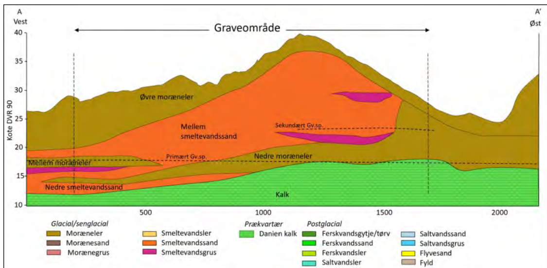
Figur 2. Geologisk tværsnit med tolket geologisk lagfølge i området C4 St. Havelse - del udlagt i 2012. Profillinjens placering fremgår af figur 3.
