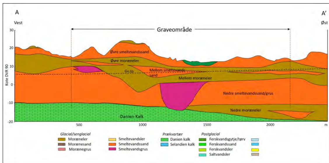
Figur 2. Geologisk tværsnit med tolket geologisk lagfølge i området D2 Sundbylille - del udlagt i 2007. Profilinjens placering fremgår af figur 3.
