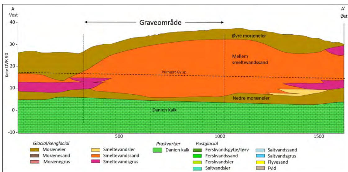
Figur 2. Geologisk tværsnit med tolket lagfølge i graveområdet L2 Ledøje Vest. Profilets placering fremgår af figur 3.
