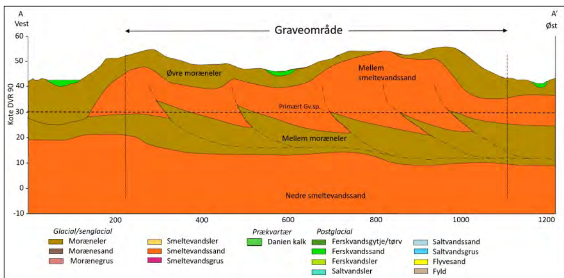
Figur 2 Geologisk tværsnit med tolket lagfølge i området A4 Kvistgård udlagt i 2012. Profilinjens placering fremgår af figur 3.
