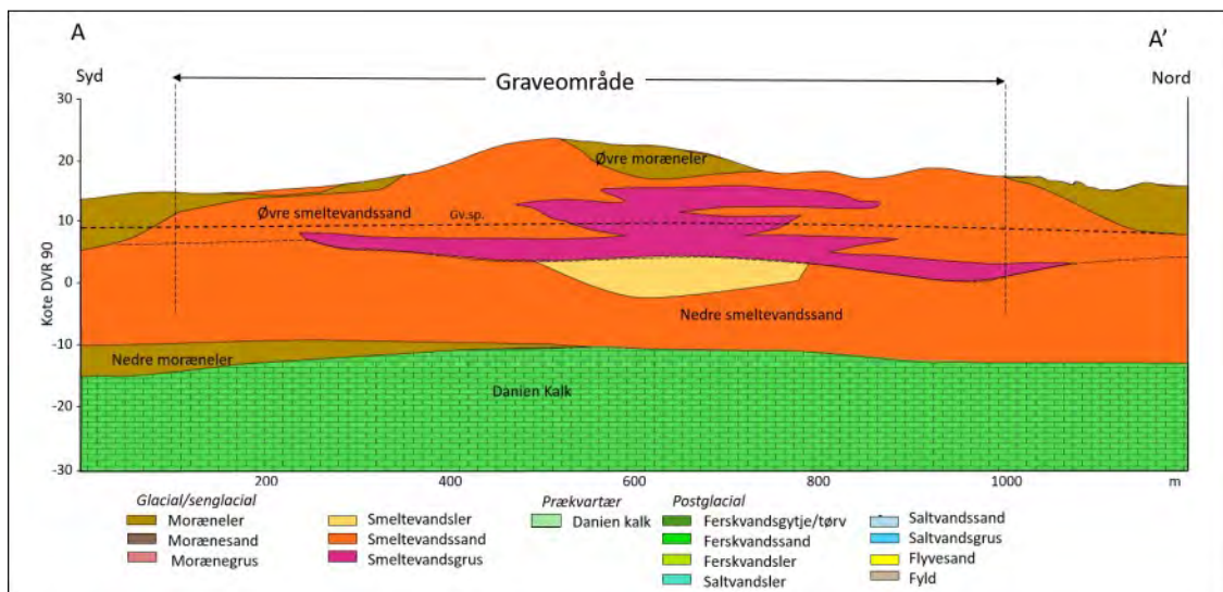
Figur 2. Geologisk tværsnit med tolket geologisk lagfølge i området D4 Lyngstrup. Profillinjens placering fremgår af figur 3.
