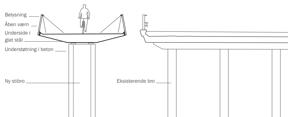
Tværsnit, Broprincip A -Stibroer, Skala 1:100
