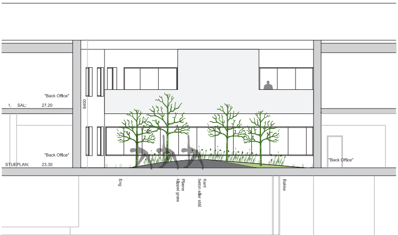
TVÆRSNIT AF AKTIVITETSHAVE - INDRE HAVERUM BYGNING 52
