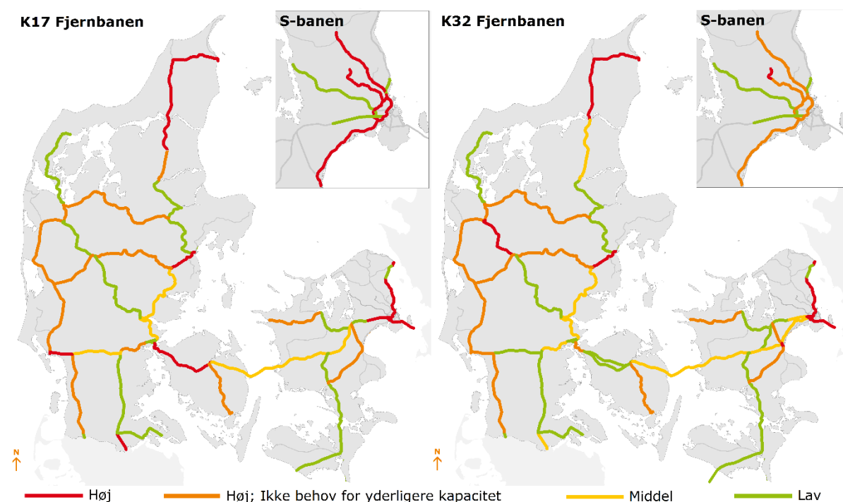
Figur 69. Kapacitetsudnyttelse 2017 og 2032
